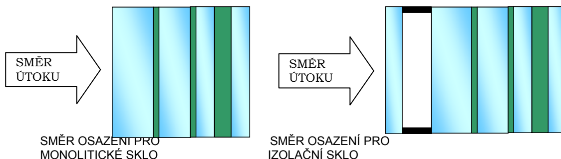
Obrázek 10 Neprůstřelné sklo použité v izolačním zasklení
