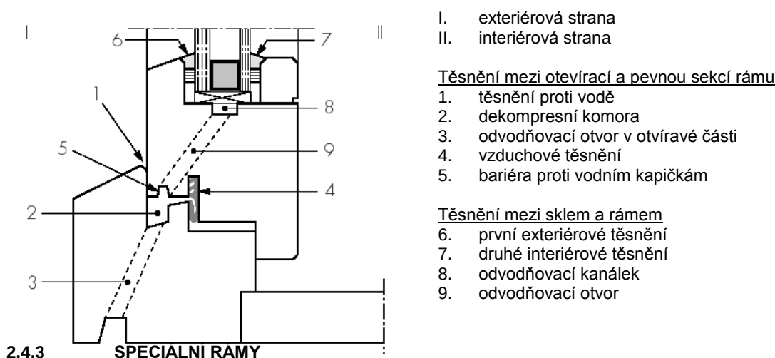
Obrázek 1 Odvodnění a utěsnění rámu
