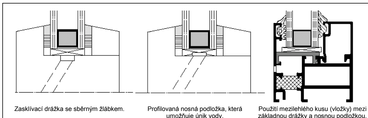
Obrázek 5 Nosné podložky mohou být přerušeny pro možnost odvodnění
