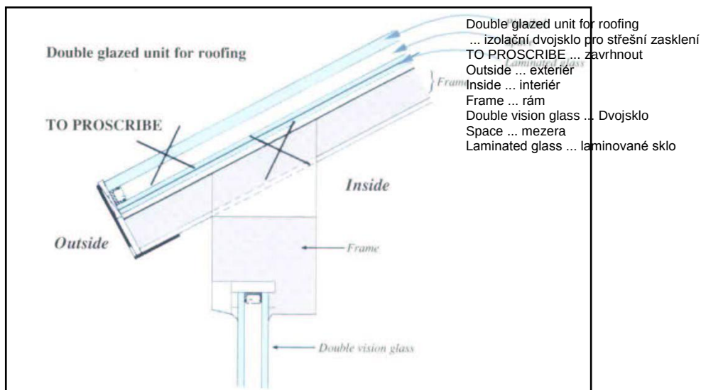
Obrázek 12 Střešní zasklení umístěné na dvou teplotách prostředí
